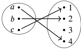
FIG. : Injective
