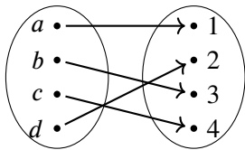
FIG. : Bijjective
