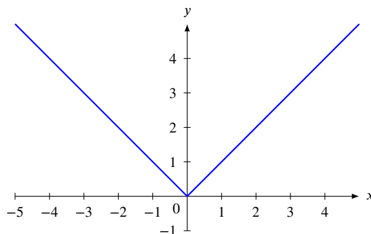
FIG. : Graphe de y = |x|
