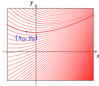
Courbes intégrales de l'EDL1 y' + y = x .
