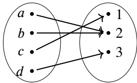
FIG. : Surjective
