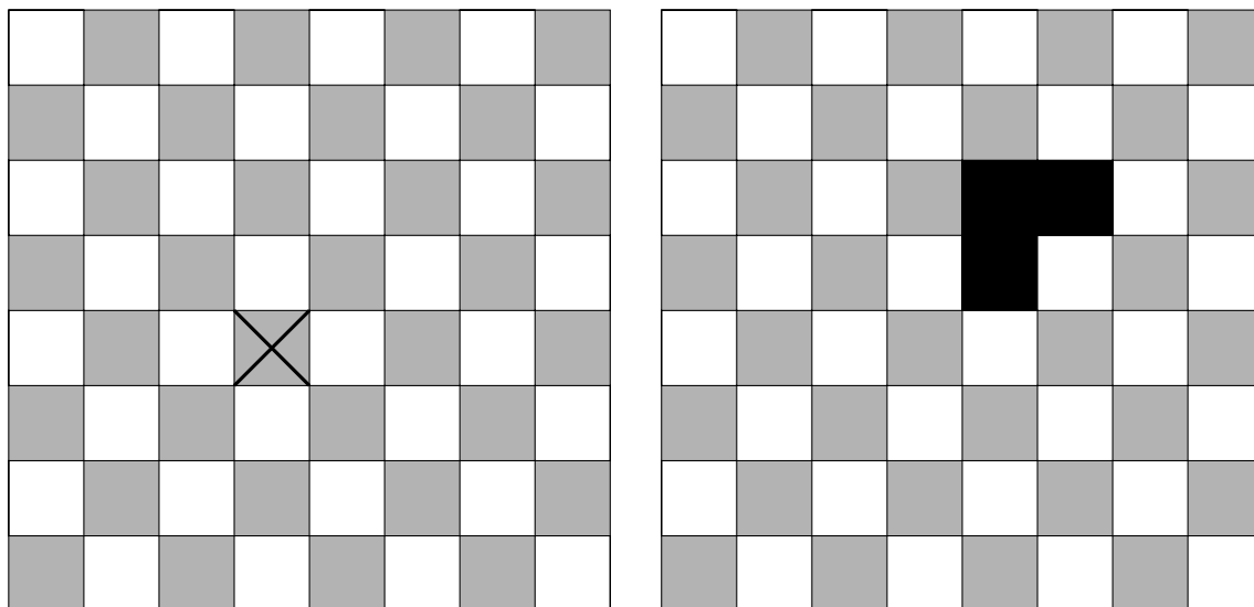
FIG. : Un damier 8 \times 8 dont une case a été retirée. FIG. : Un tromino en forme de L sur un damier.
